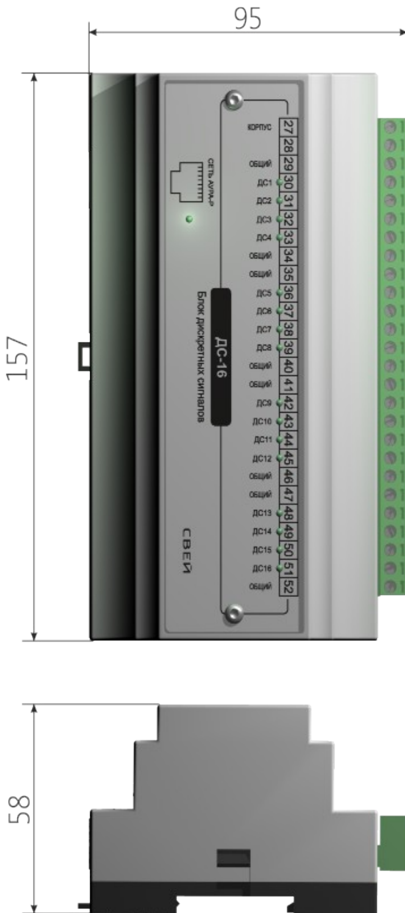
Рисунок 85: Габаритные размеры блока дискретных сигналов ДС-16
